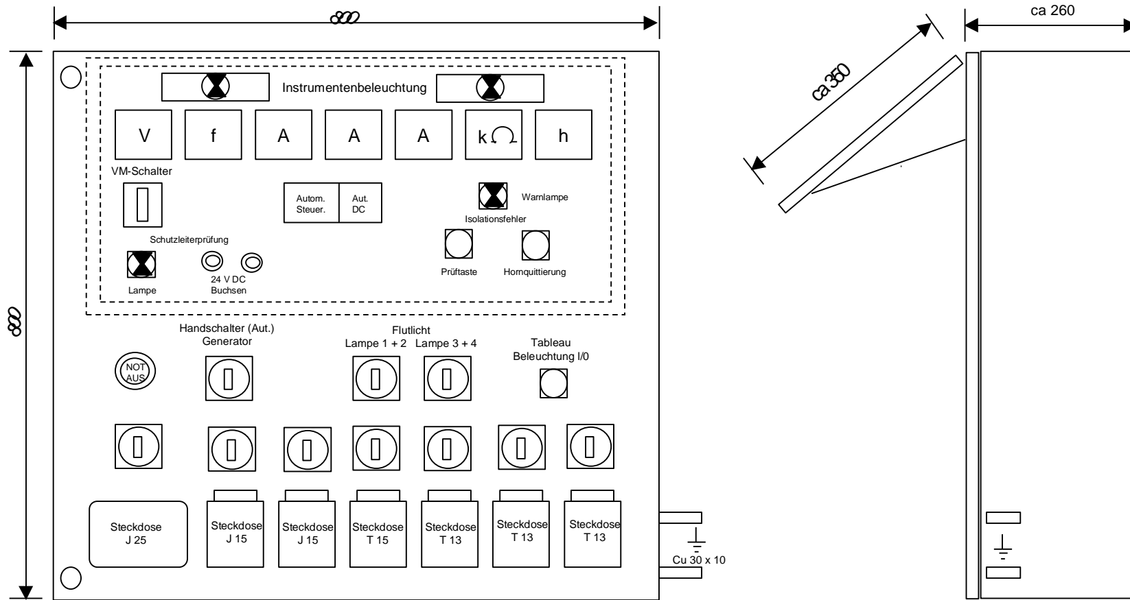
Schaltschrank Steckdosentableau
